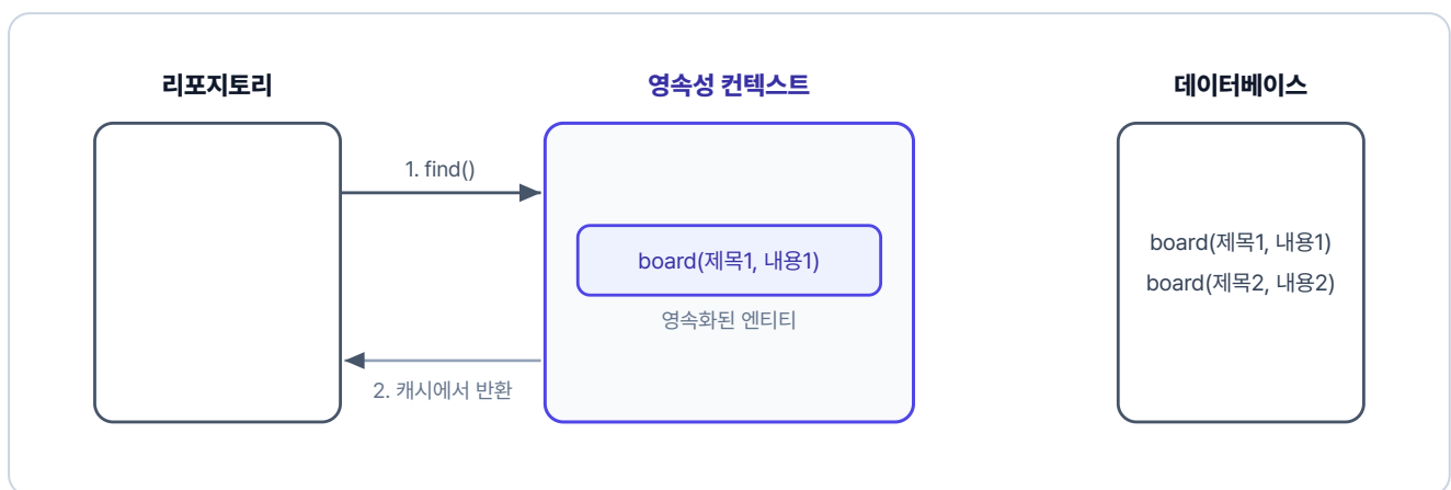
그림 2-21. 캐시 조회
